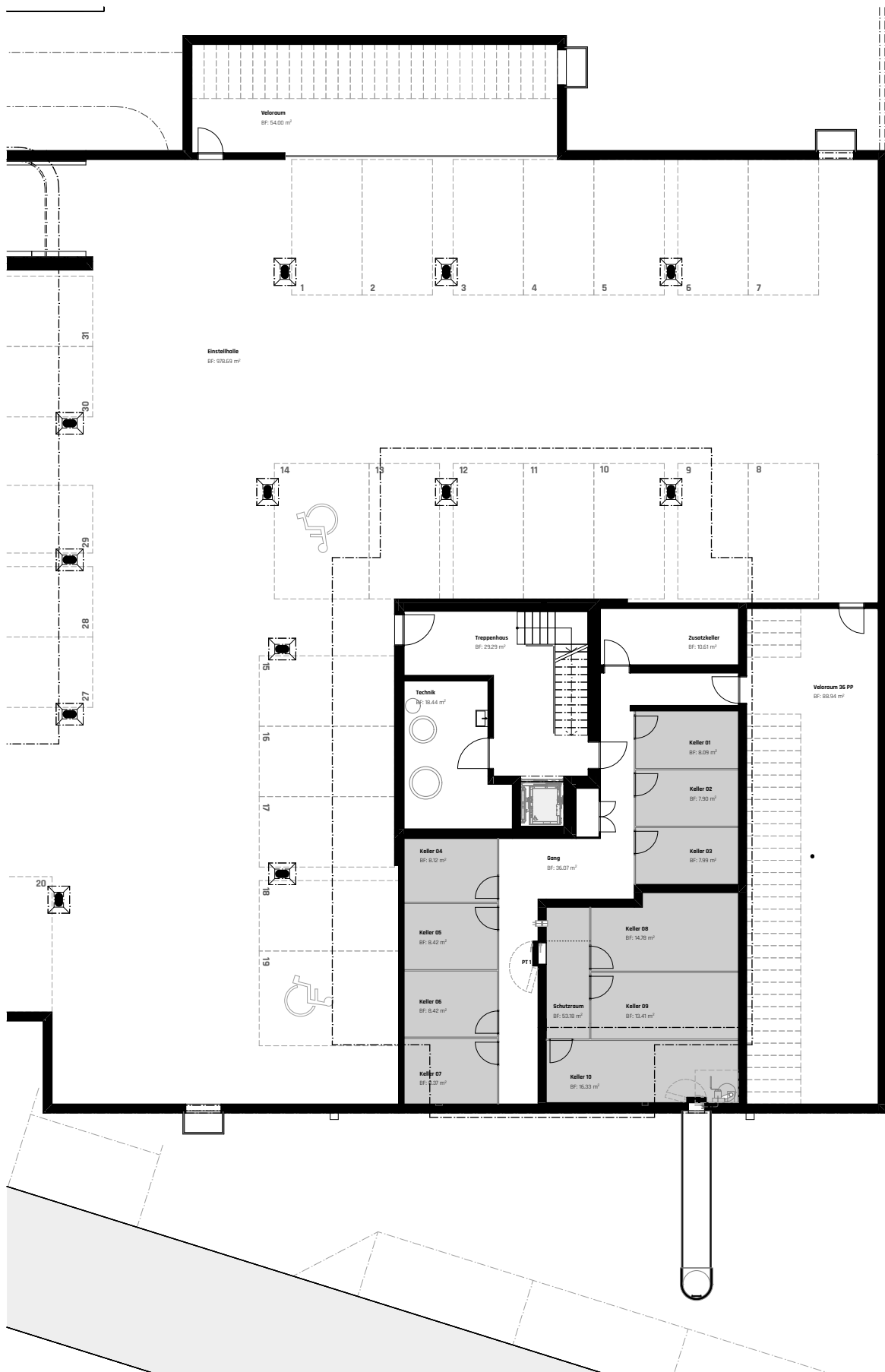
Haus B - Untergeschoss / Mst. 1:150
