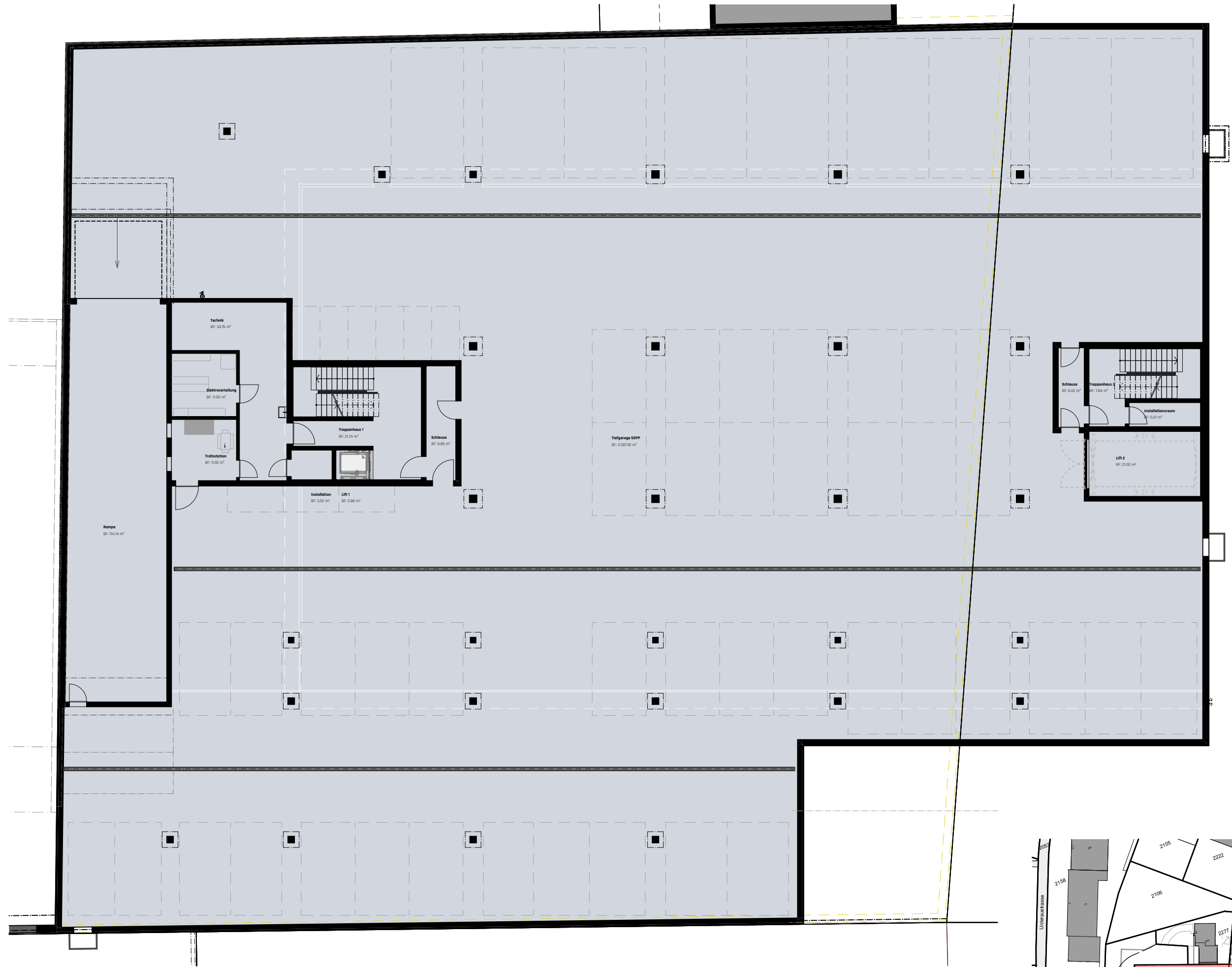
Halle 3 - Untergeschoss / Mst. 1:200
