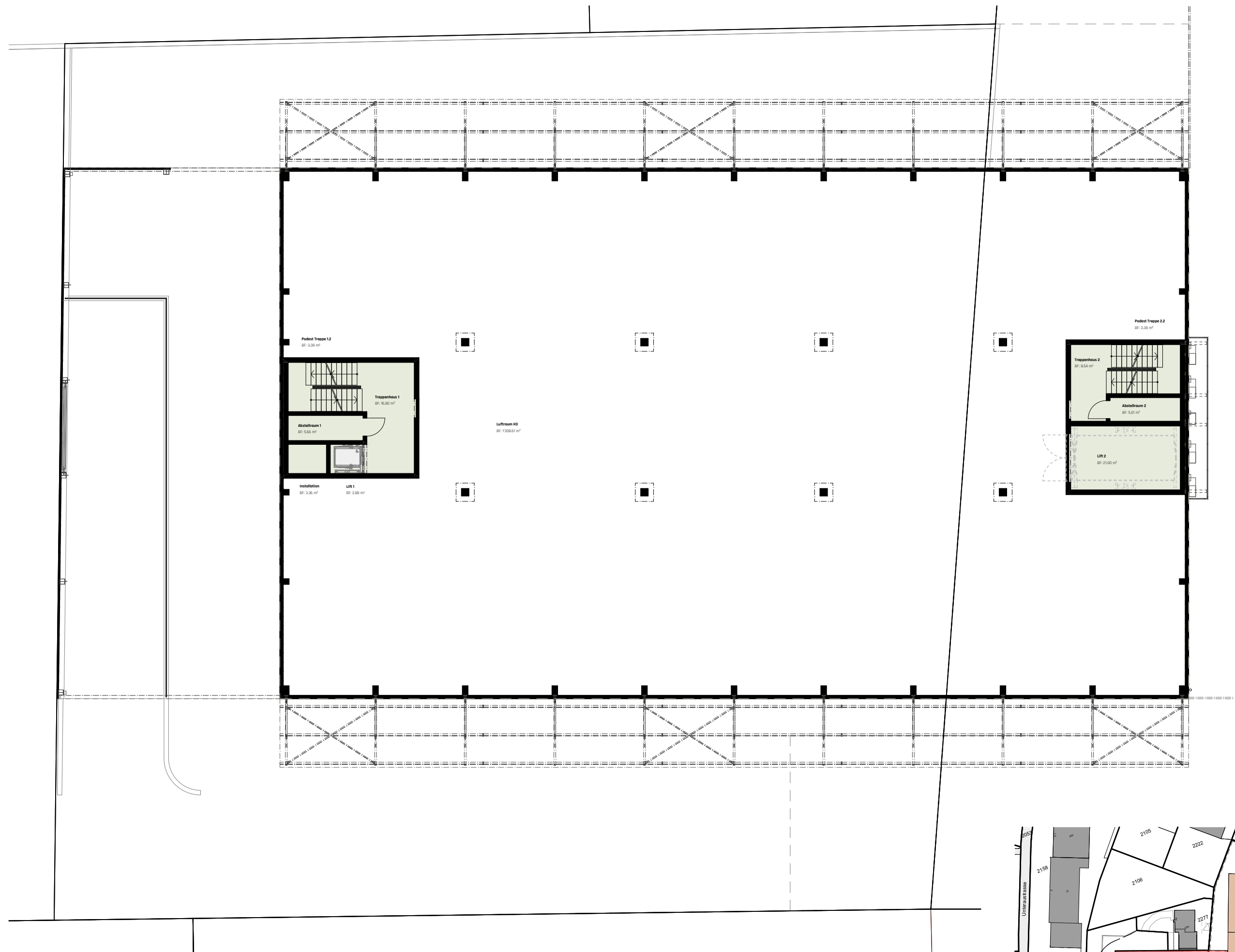
Halle 3 - 1. Obergeschoss (Luftraum) / Mst. 1:200
