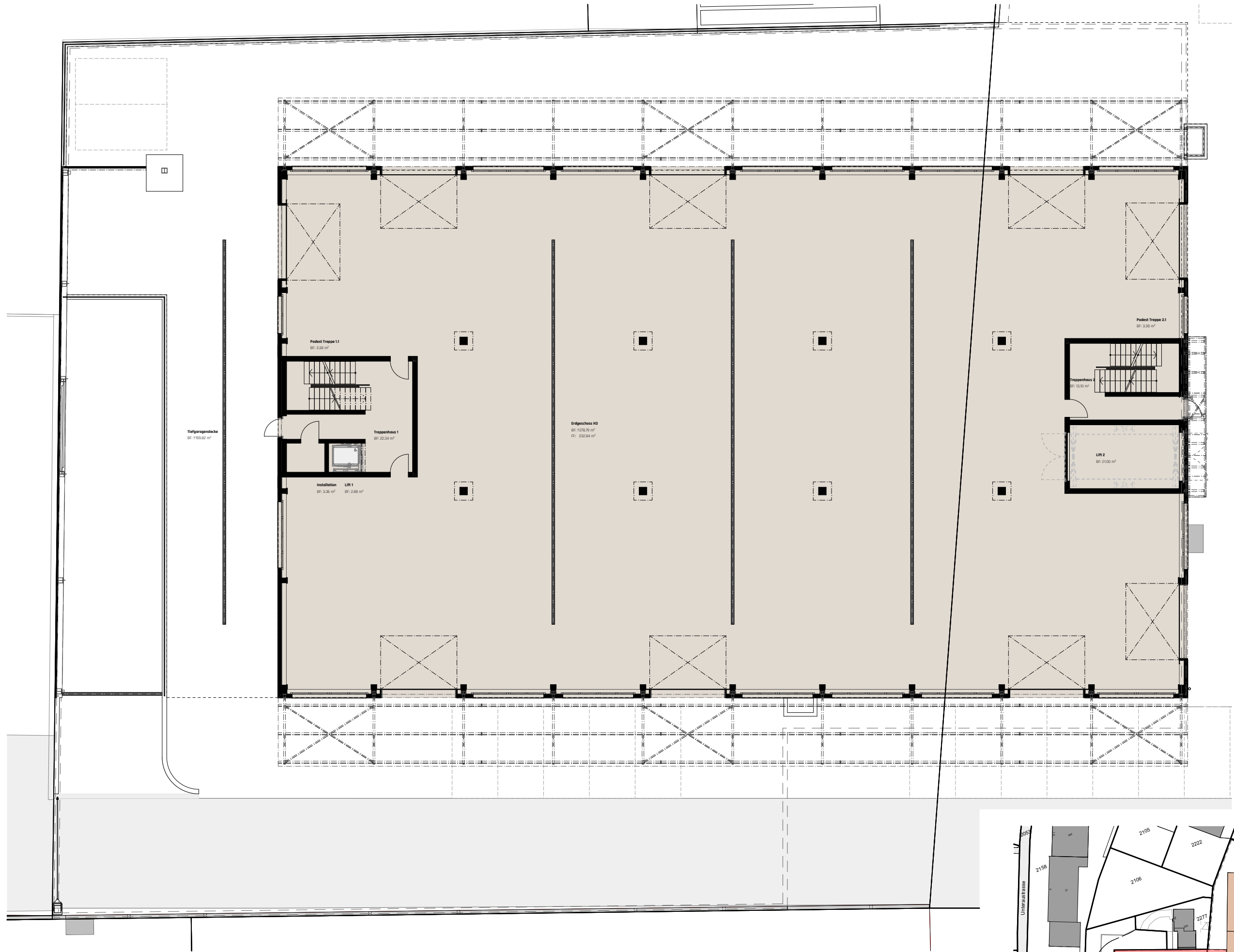
Halle 3 - Erdgeschoss / Mst. 1:200
