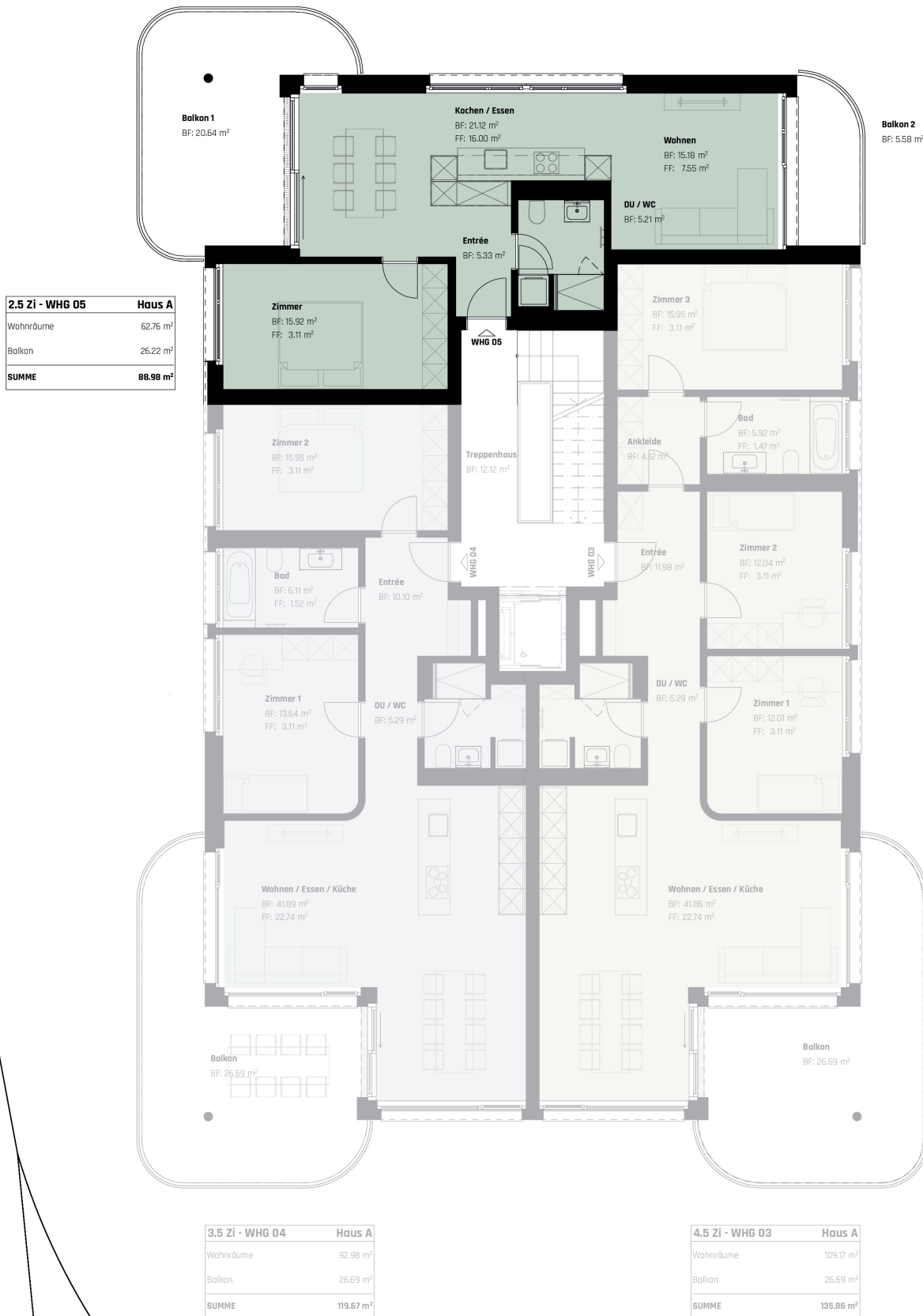
Haus A - 1. Obergeschoss / Mst. 1:100
